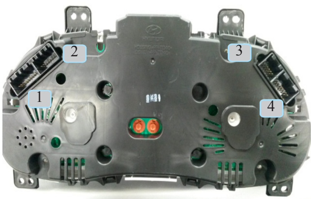
Фото 3.4. Нумерация разъёмов панели приборов
