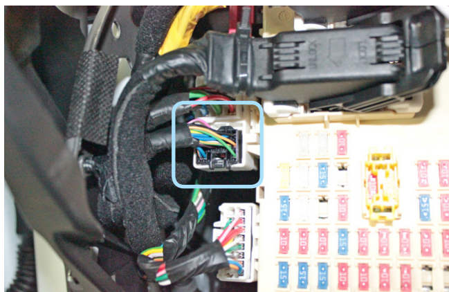
Фото 3.17. Местоположение разъёма
