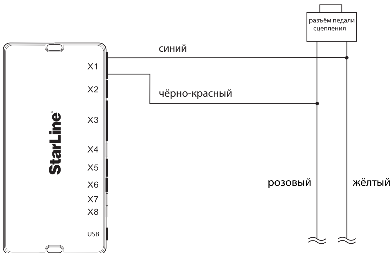
Схема 2. Имитация нажатия педали сцепления
