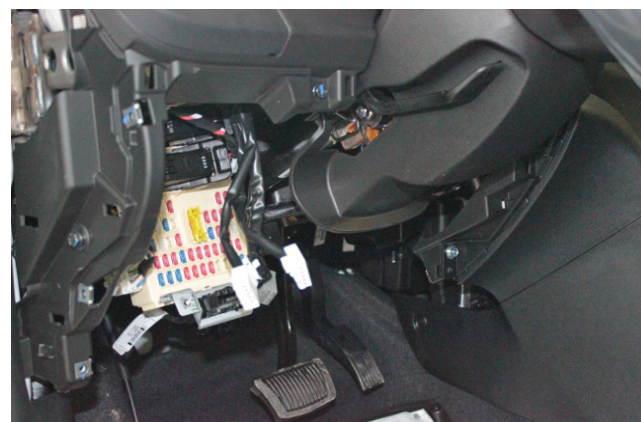
Фото 1.6. Пластиковая накладка под рулевой колонкой снята
