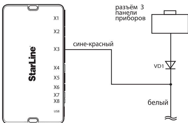
Схема 1. Подключение контроля стояночного тормоза
