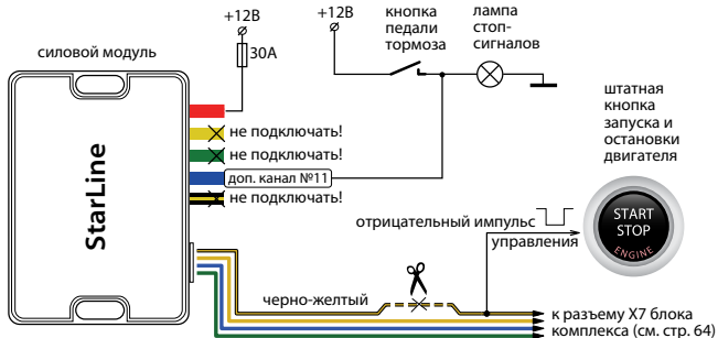
Схема 2: слаботочное управление кнопкой «старт-стоп»
