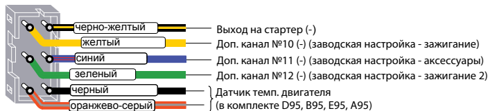
разъем Х7 (слаботочные выходы)
