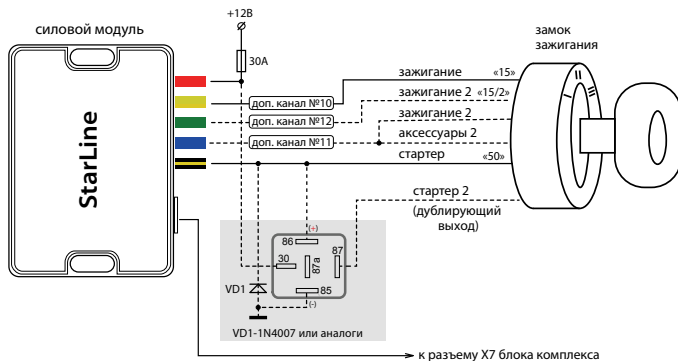
разъем Х7 (слаботочные выходы)
