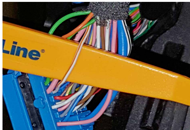
Фото 8.2. Шина данных штатного иммобилайзера (бело-оранжевый)
