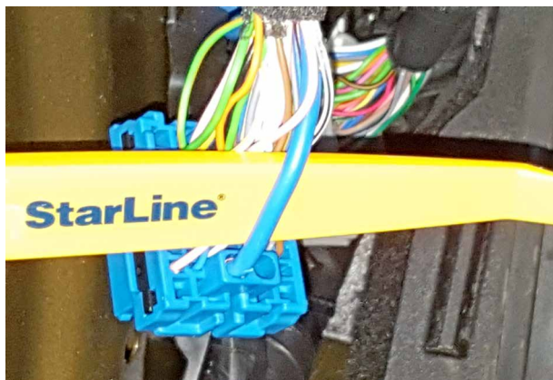
Фото 9.1. Зажигание 1 (синий)
