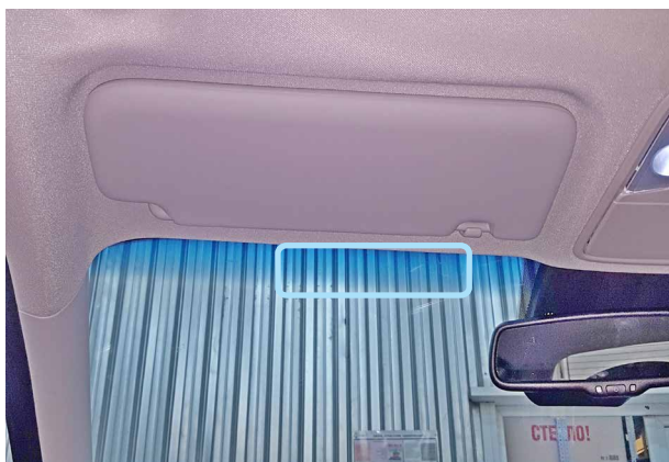
Фото 3.1. Возможное место установки антенного модуля
