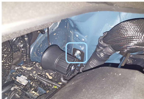
Фото 4.2. Крепление сирены
