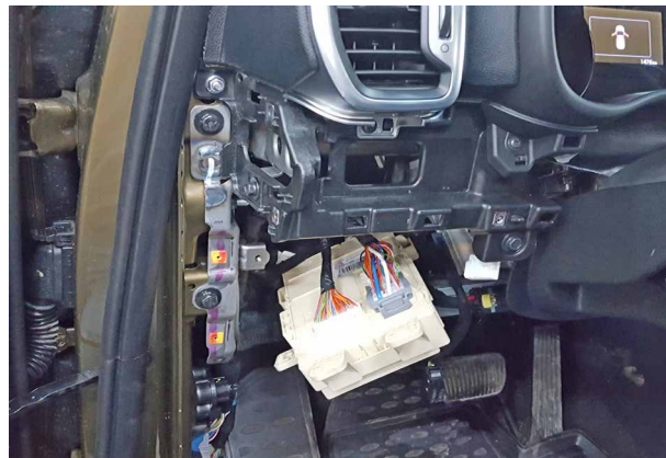
Фото 2.4. Монтажный блок предохранителей снят
