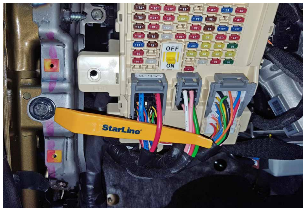
Фото 10. Питание +12В (красный)
