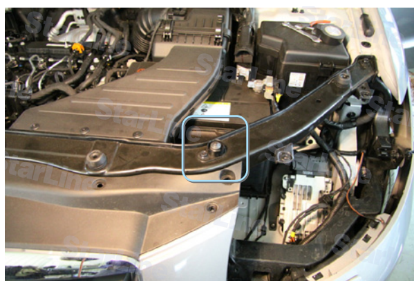
Фото 6.5. Концевик капота
