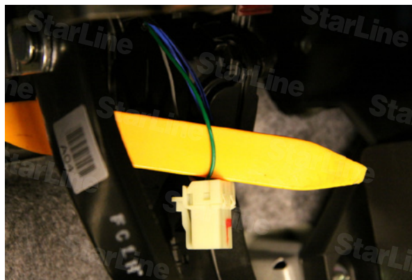
Фото 14.2. Стоп-сигнал (зеленый)
