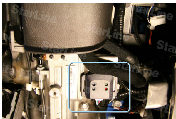
Фото 8.5. Датчик удара
