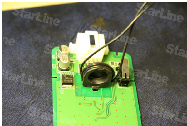
Фото 17.1. Плата с катушкой
