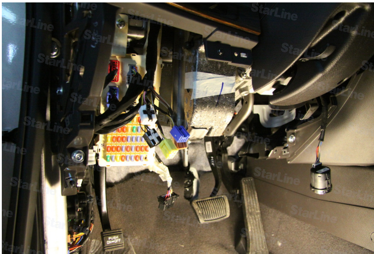
Фото 2. Общий вид
