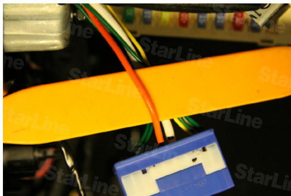
Фото 16.2. Зажигание (IGN-оранжевый)
