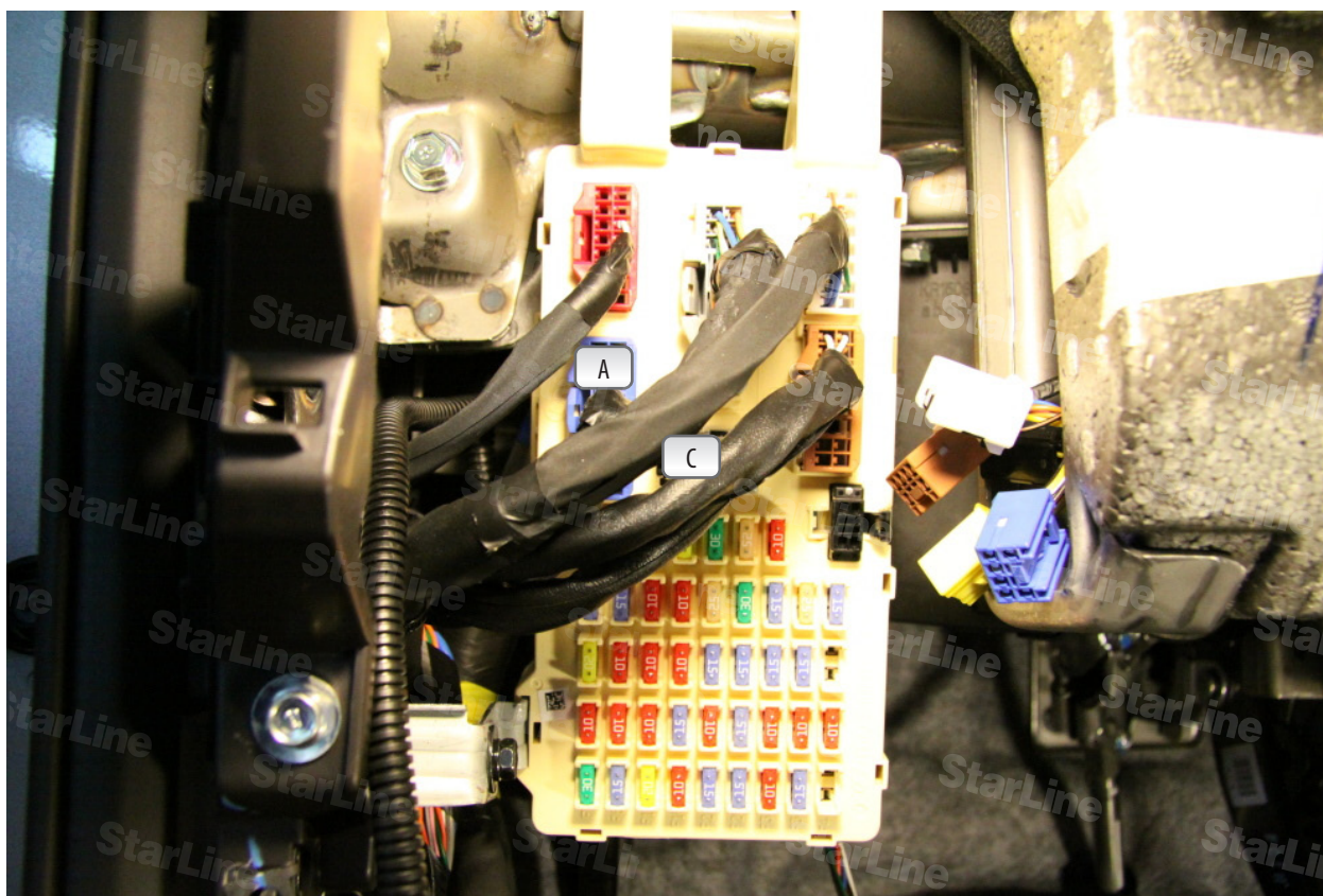
Фото 16.1. Блок BCM
