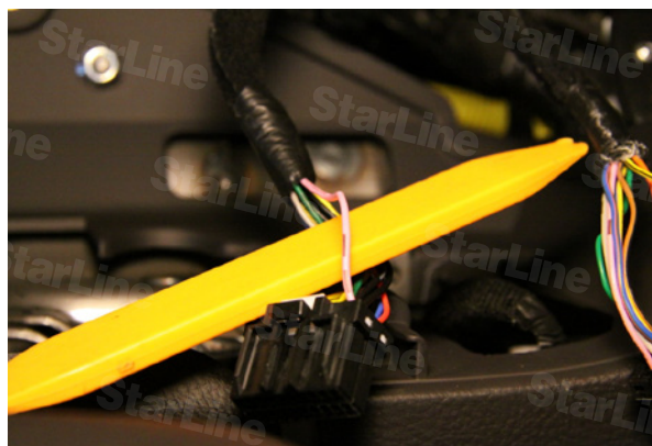
Фото 11.2. Поворотник (розовый)
