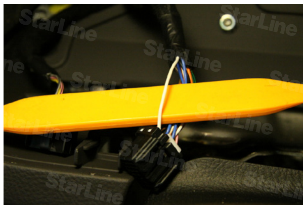
Фото 11.1. Поворотник (белый)
